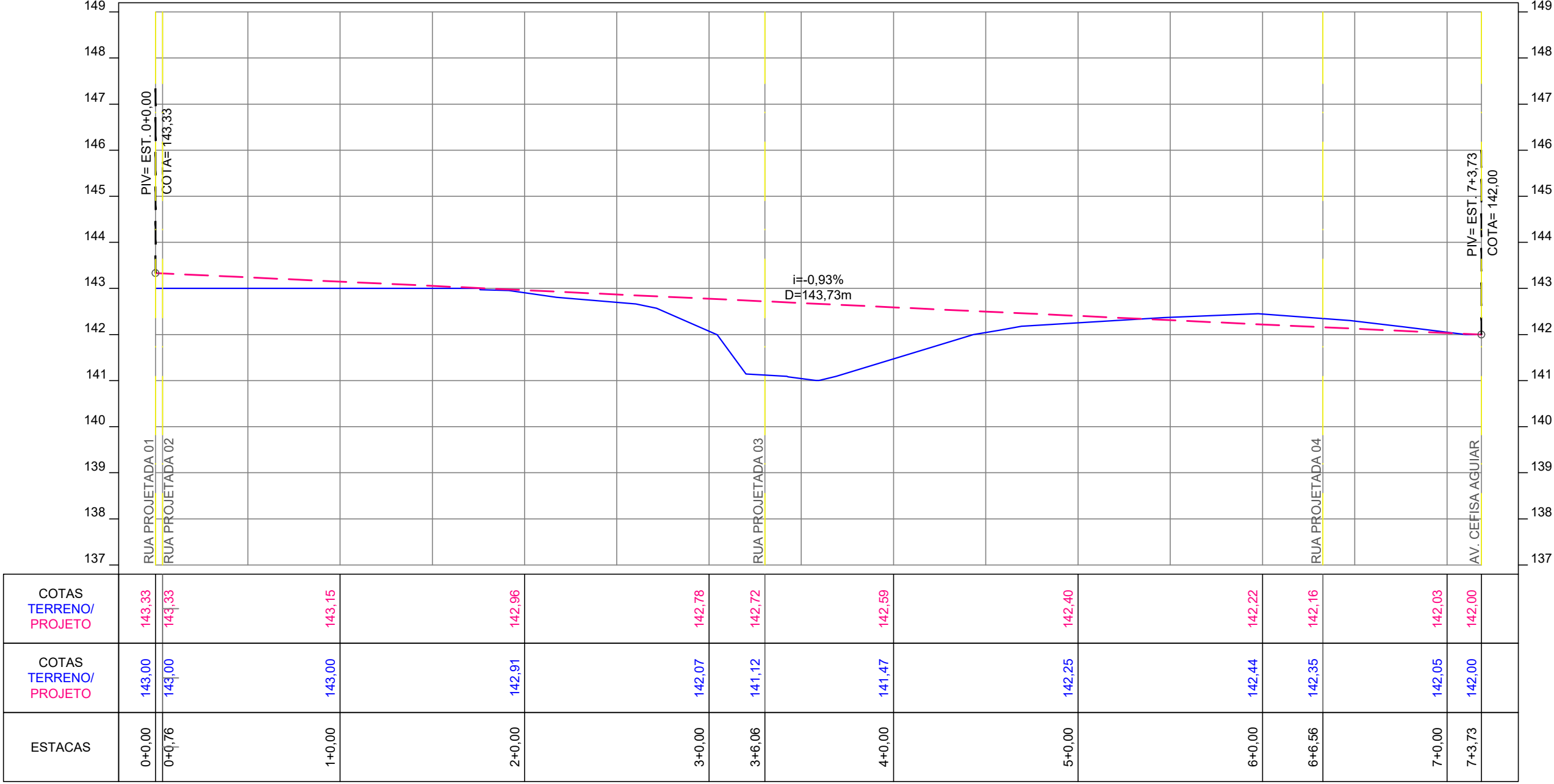
PERFIL LONGITUDINAL - RUA PROJETADA 06 Esc.: H=1/500 - V=1/100
