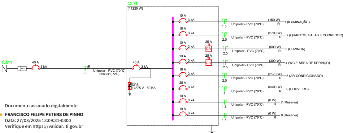
3 QUADRO UNIFILAR QD1 ESCALA: 1:100
