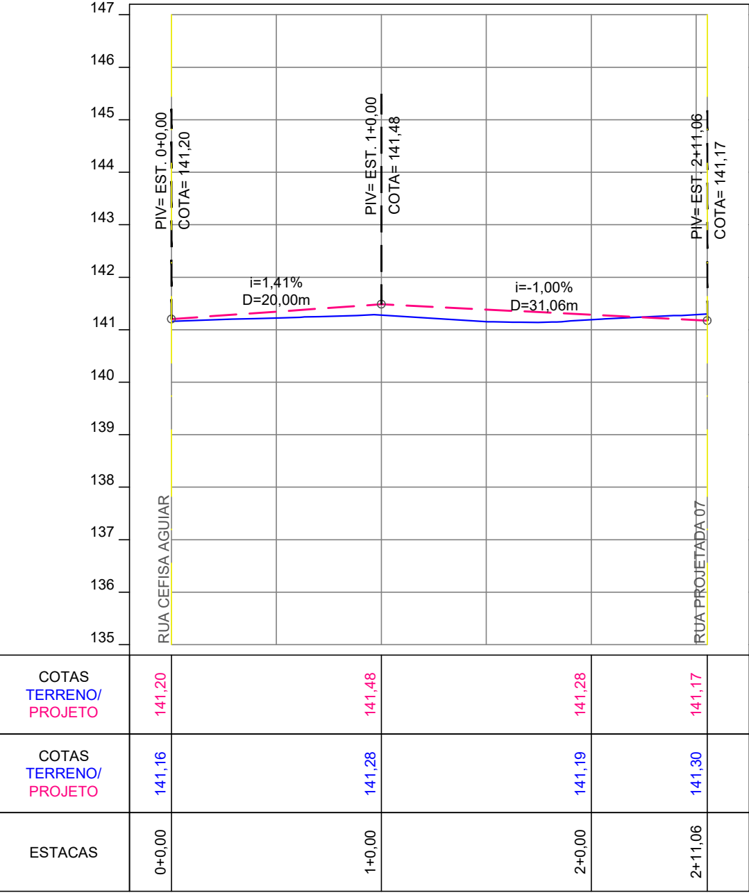
PERFIL LONGITUDINAL - RUA PROJETADA 05 Esc.: H=1/500 - V=1/100
