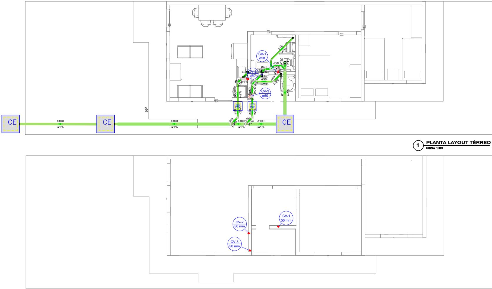
2 PLANTA LAYOUT COBERTA ESCALA 1:100
