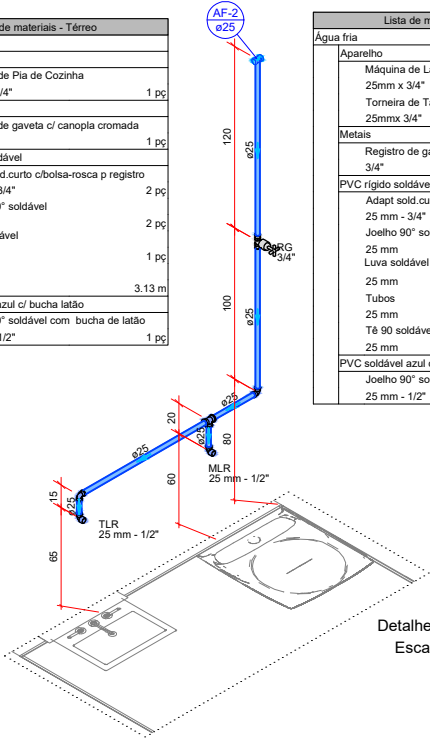
Detalhe HID-2 Escala 1:50
