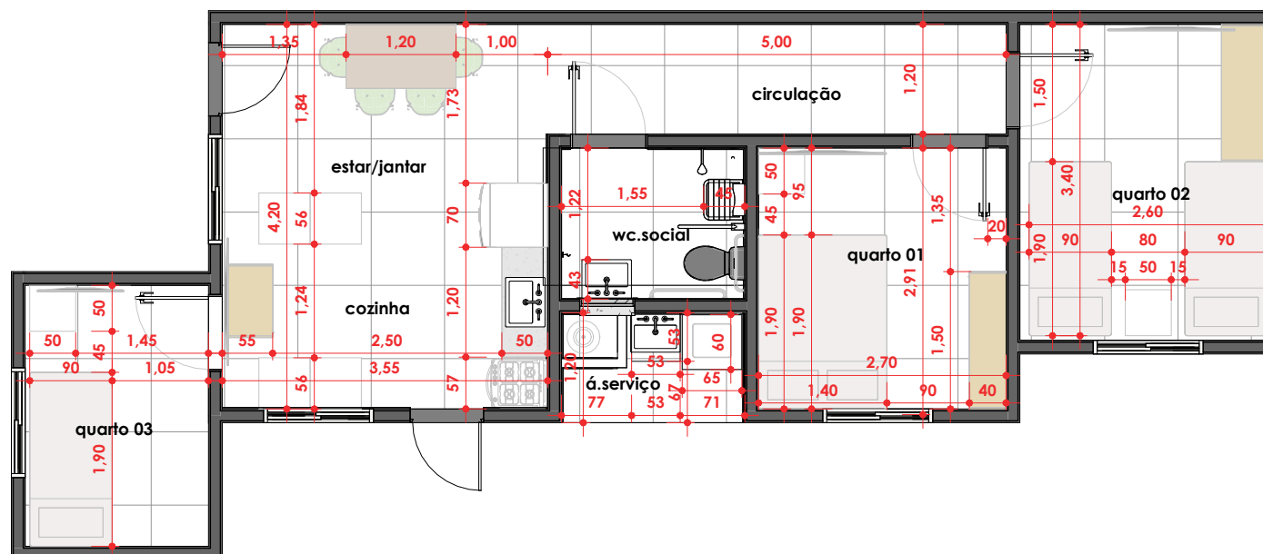
Térreo - Layout de Mobiliários e Equipamentos
