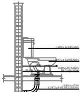
DET. GEN. VASO SANITÁRIO SEM ESCALA
