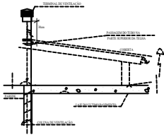
DET.VENTILAÇÃO SEM ESCALA
