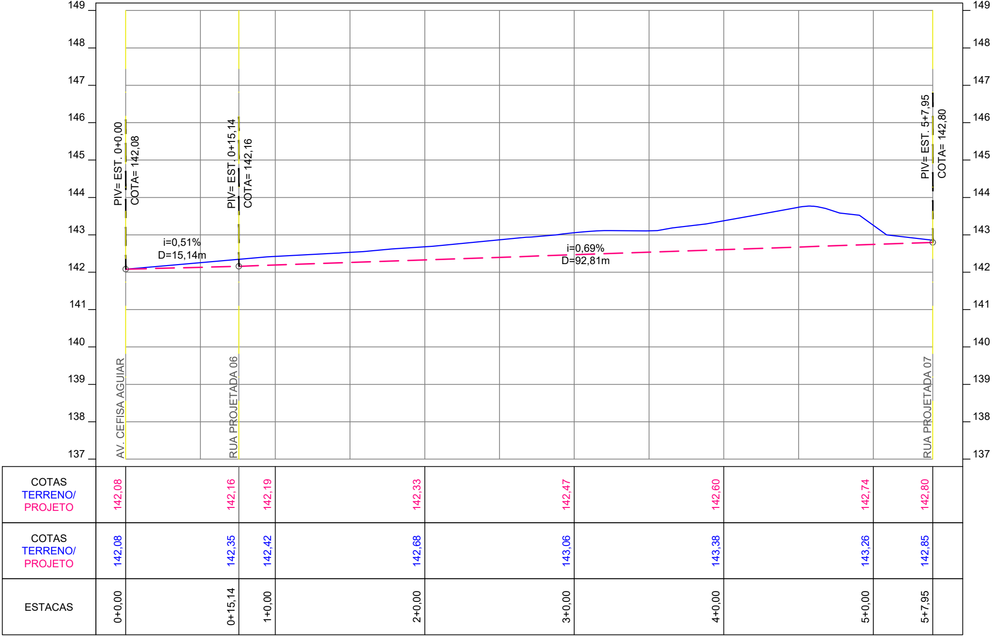
PERFIL LONGITUDINAL - RUA PROJETADA 04 Esc.: H=1/500 - V=1/100
