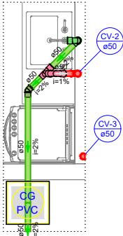
Detalhe SAN-1 Escala 1:50
