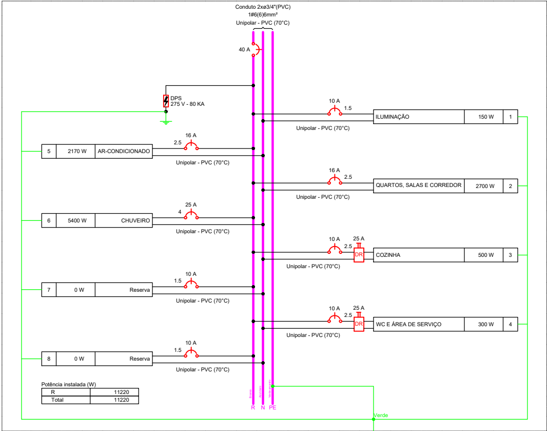
2 QUADRO MULTIFILAR QD1 ESCALA: 1:100
