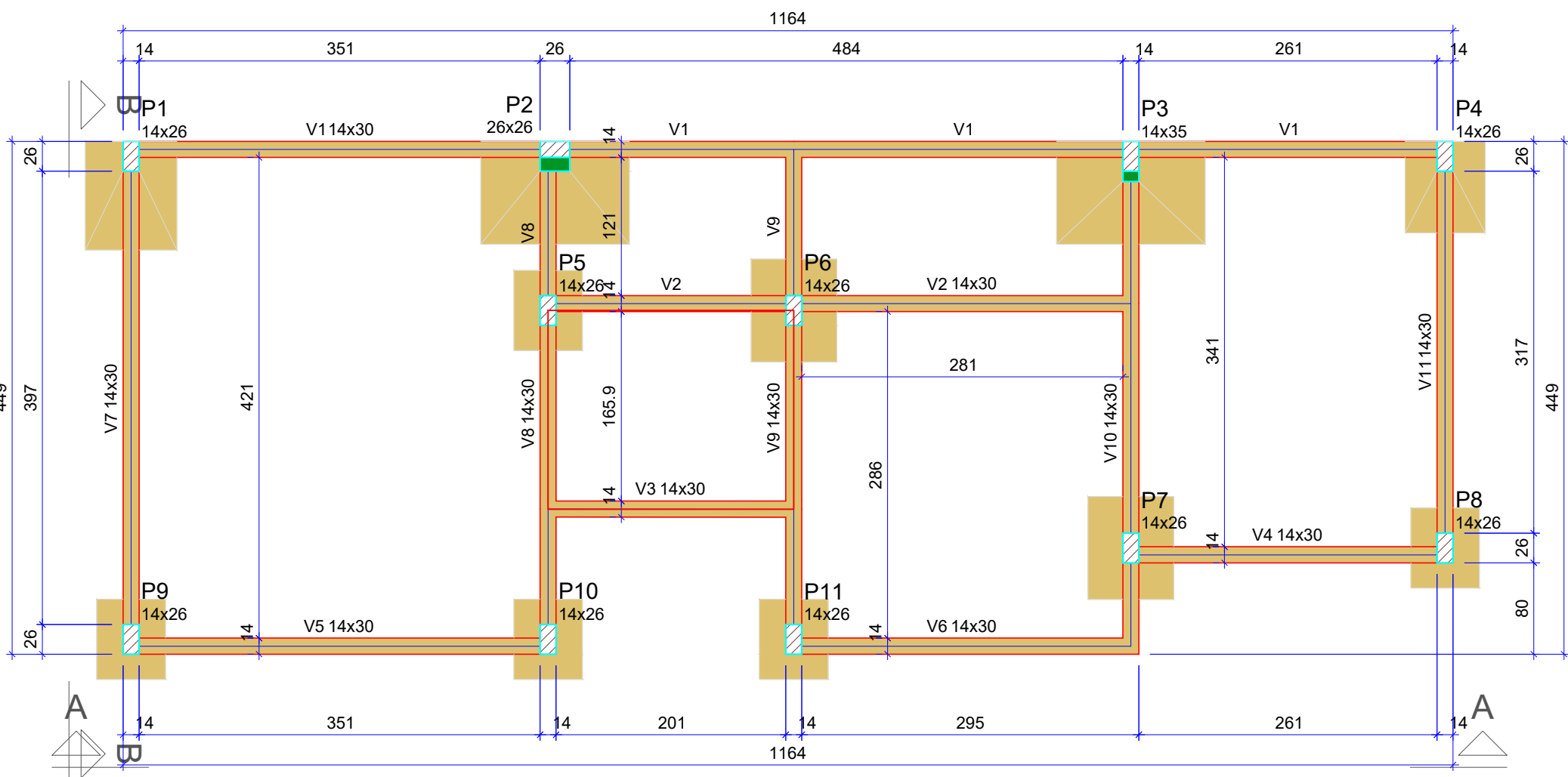
Forma do pavimento Baldrame - Nível 0 cm (Nível 0) escala 1:50
